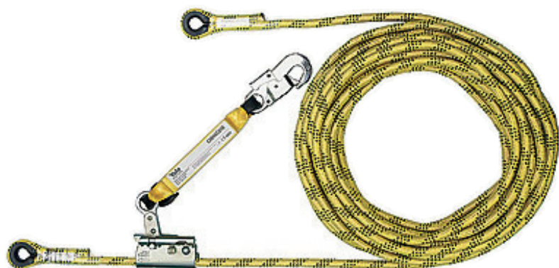
חבל עיגון לעבודה בגובה (קו חיים) לפי תקן EN-352-2 אורך 20/15 מטר מק"ט: 10-116-11
